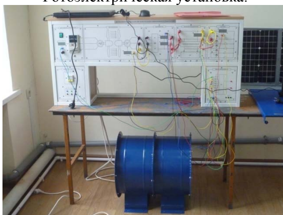
Ветроэнергетическая установка с асинхронным генератором.
